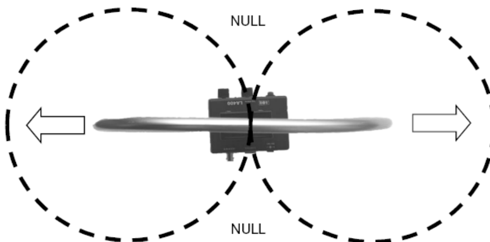
LA-400 – radiazione orizzontale
