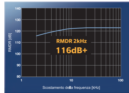
Gamma dinamica reciproca al mixer della banda da 14 MHz (RMDR)
